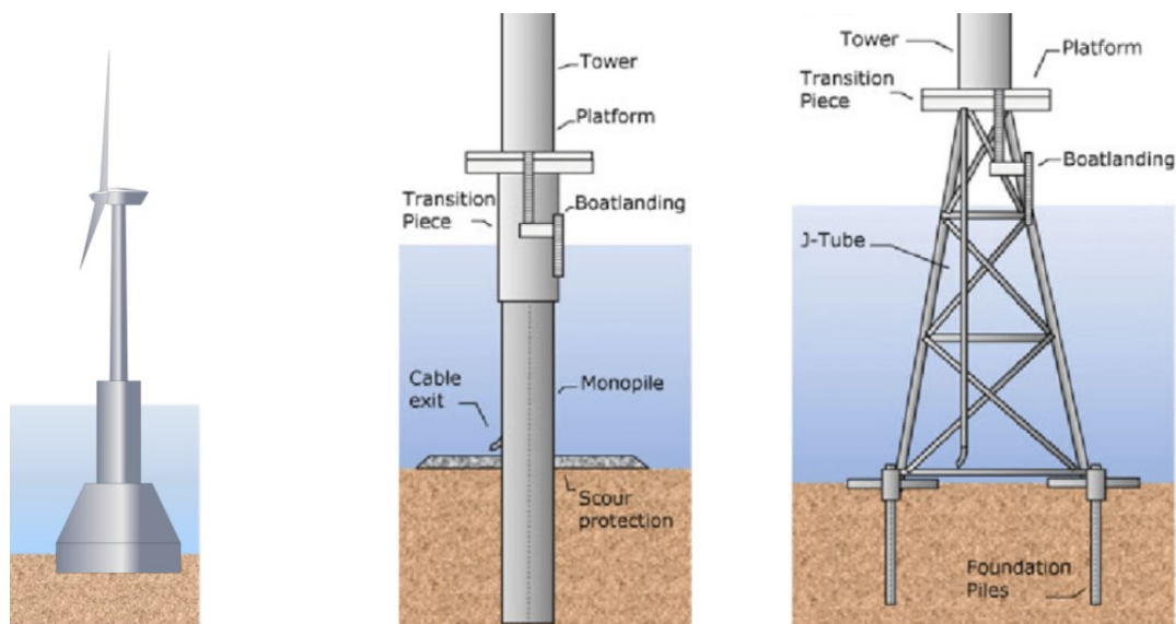
Rysunek 3.4. Poglądowe rysunki poszczególnych typów fundamentów (od lewej): grawitacyjny; monopilewy; kratownicowy (źródło: https://www.obayashi.co.jp/chronicle/130th/en/archives/chapter4_1_5.html# oraz: https://www.researchgate.net/figure/Three-types-of-turbine-foundations-Monopile-a-jacket-b-and-gravity-based-c_fig2_315874967 )
