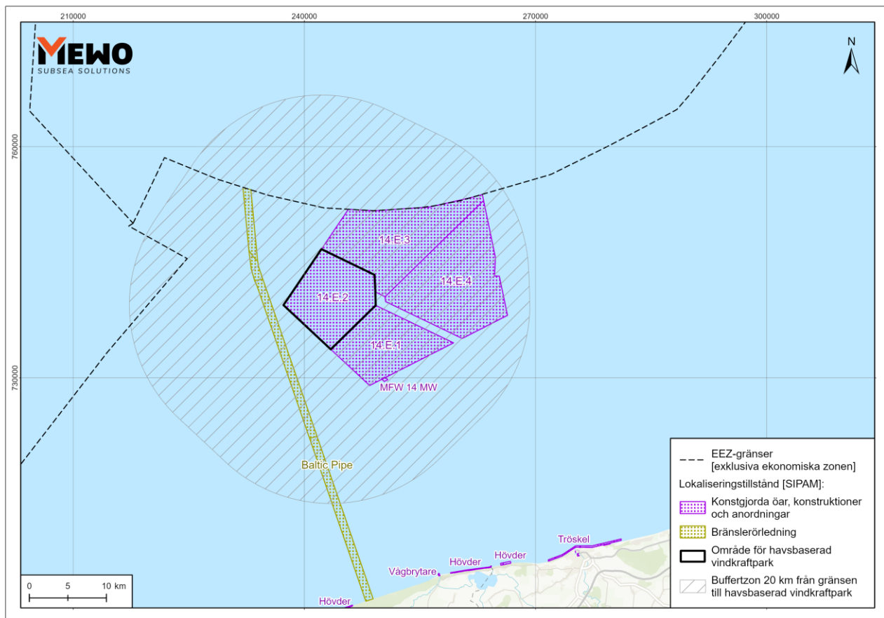
Figur 2.1. Lokalisering av området för havsbaserad vindkraftpark HAVV 14.E.2 och angränsande områden för havsbaserad vindkraftpark som omfattas av tillstånd för uppförande av konstgjorda öar och konstruktioner utfärdade av infrastrukturministern (källa: egen bearbetning baserad på data från SIPAM)
