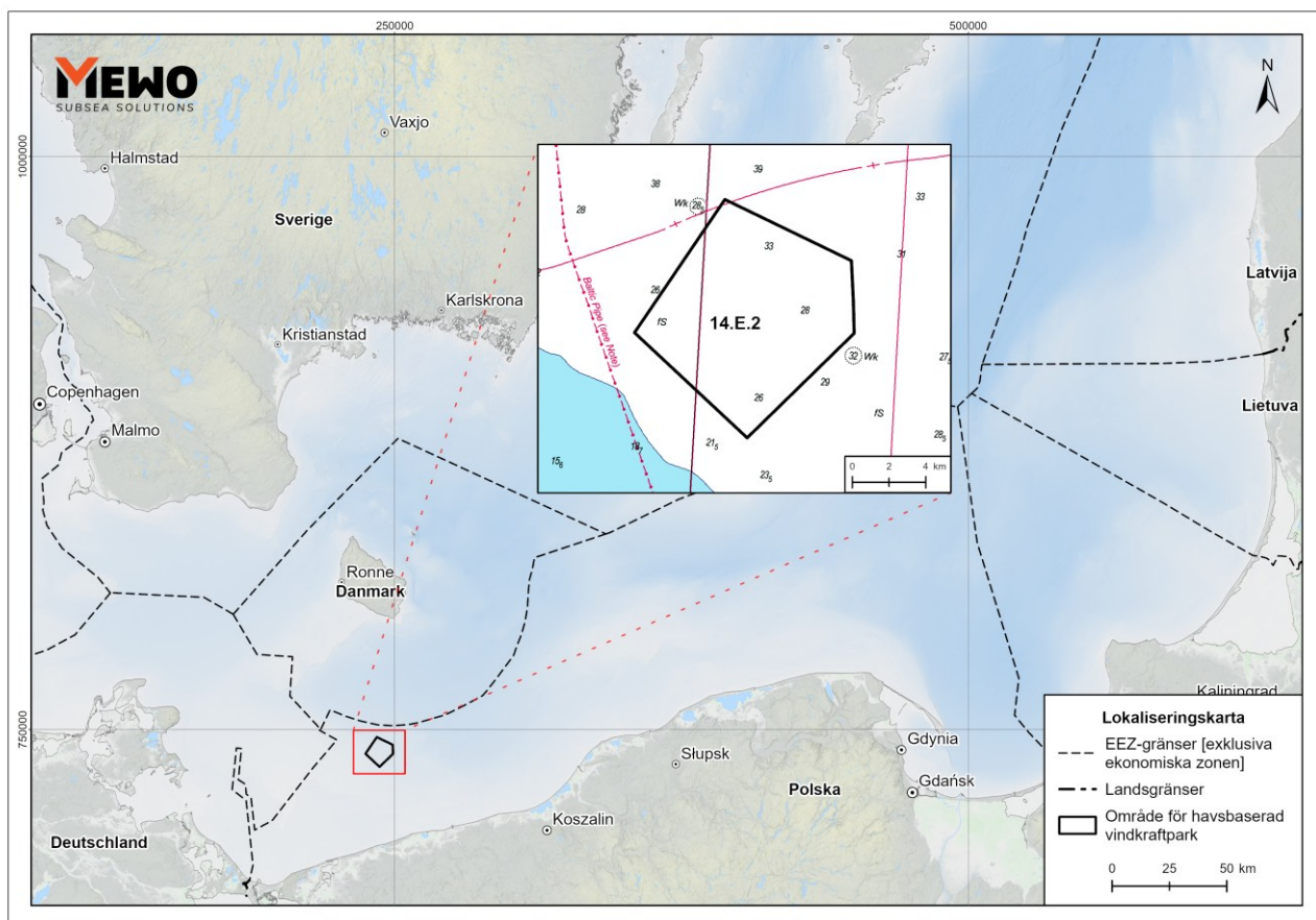
Figur 1.1. Lokalisering av området för havsbaserad vindkraftpark HAVV 14.E.2 i polska havsområden (källa: egen bearbetning)
