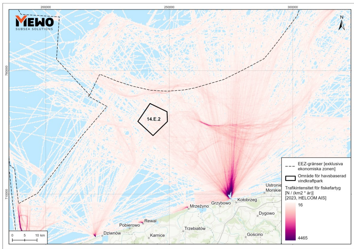
Figur 2.4. Lokalisering av området för havsbaserad vindkraftpark HAVV 14.E.2 i förhållande till fiskefartygens användning av havsområdet. AIS-data – genomsnitt för 2023 (källa: egen bearbetning baserad på data från EMODnet)
