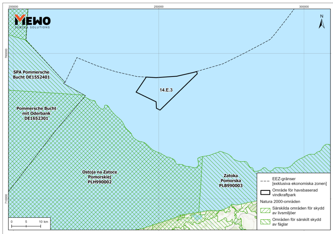
Figur 9.1. Lokalisering av området för havsbaserad vindkraftpark HAVV 14.E.3 i förhållande till områden som omfattas av skydd enligt lagen av den 16 april 2004 om naturskydd (jfr. Polens officiella tidning från 2022 p. 916 med senare ändringar). (källa: egen bearbetning)
