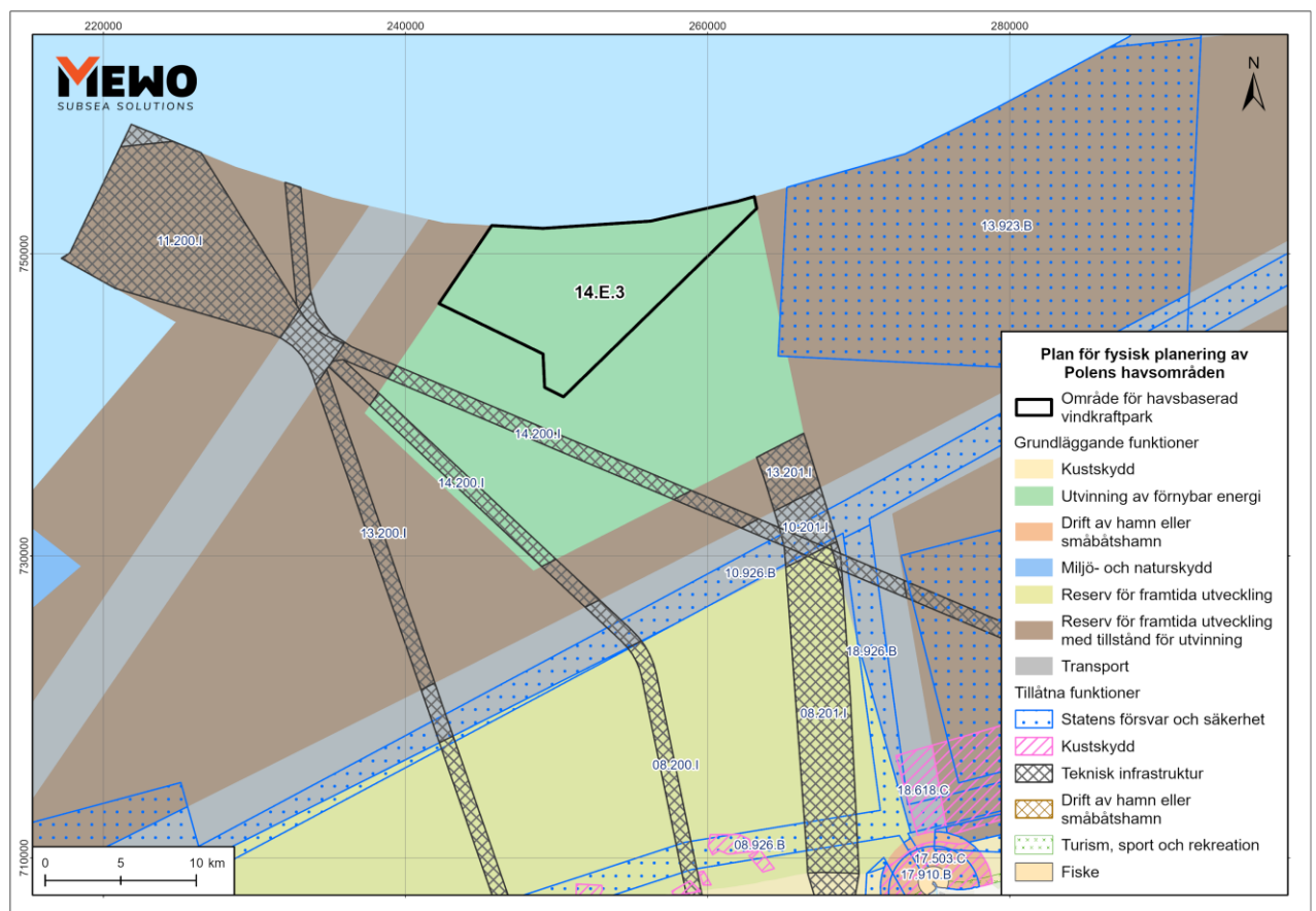
Figur 1.2. Lokalisering av området för havsbaserad vindkraftpark HAVV 14.E.3 i förhållande till vattenområden och delvattenområden enligt polska planeringen av havsområden (källa: egen bearbetning baserad på rumsliga data från Sjöförvaltningens system för rumslig information (SIPAM) [System Informacji Przestrzennej Administracji Morskiej])
