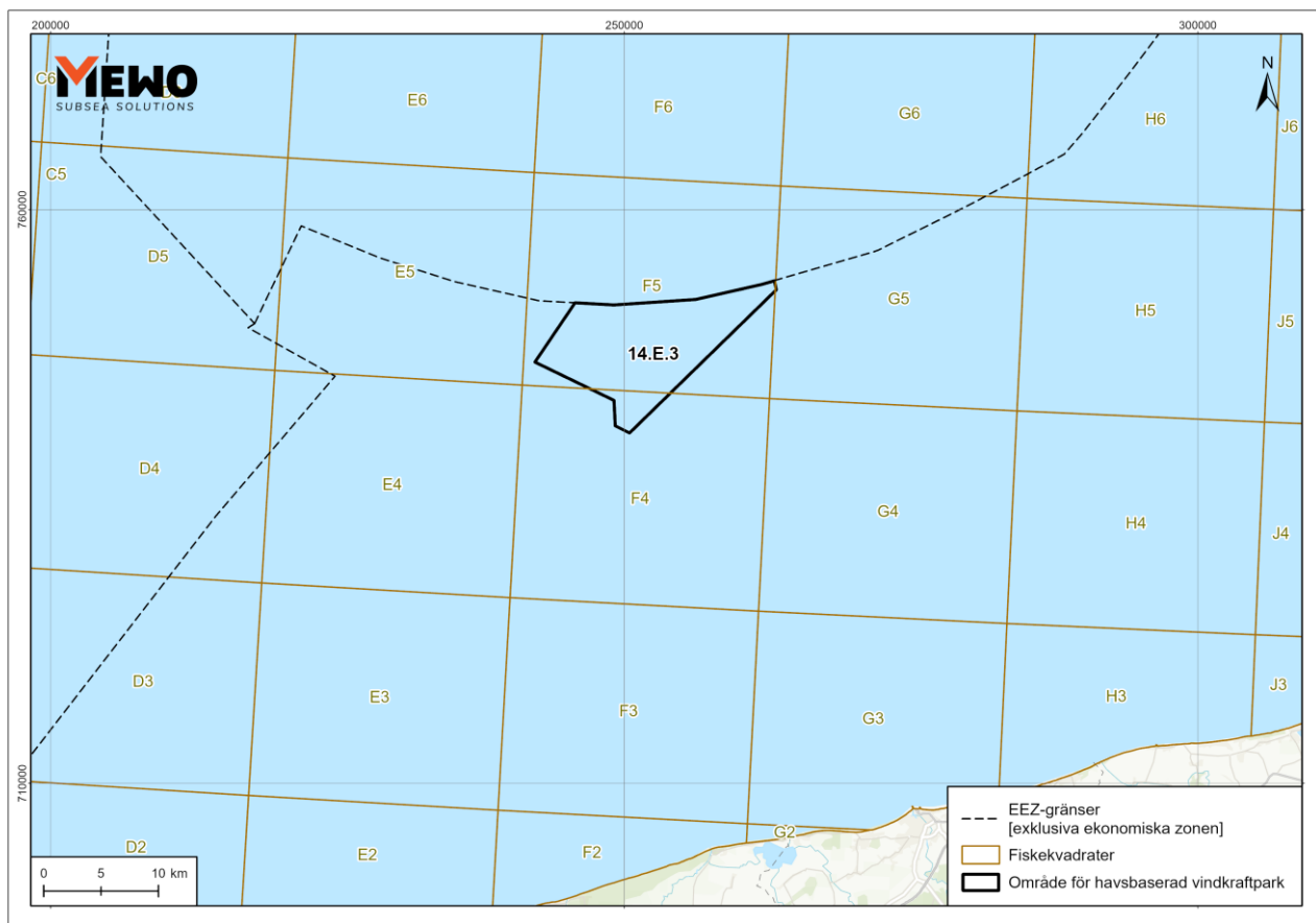
Figur 2.2. Lokalisering av området för havsbaserad vindkraftpark HAVV 14.E.3 i förhållande till fiskekvadrater (källa: egen bearbetning baserad på data från Fiskeribevakningscentralen vid Ministeriet för jordbruk och landsbygdsutveckling)
