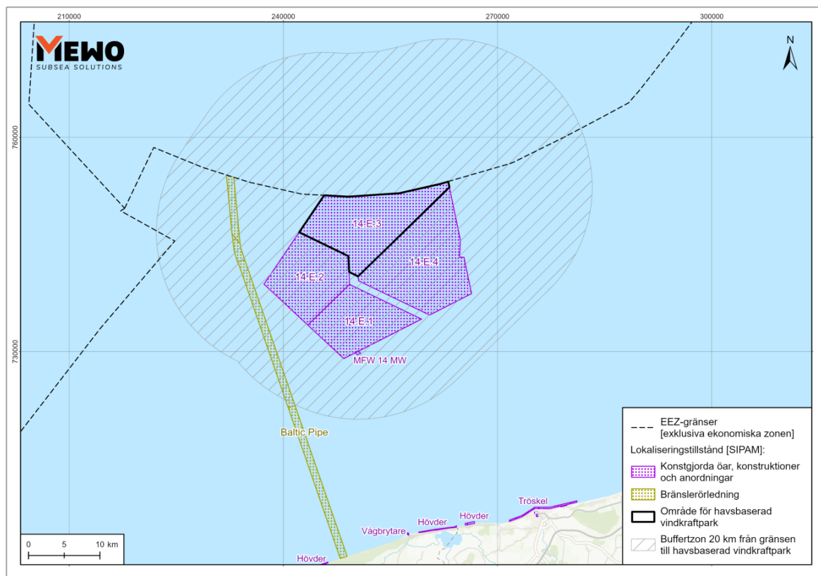
Figur 10.1. Lokalisering av projekt som planeras utanför området för HAVV 14.E.3, som kan komma att påverkas av projektet eller vars påverkan kan ackumuleras med påverkan från HAVV 14.E.3 (källa: egen bearbetning baserad på data från Sjöförvaltningens system för rumslig information)
