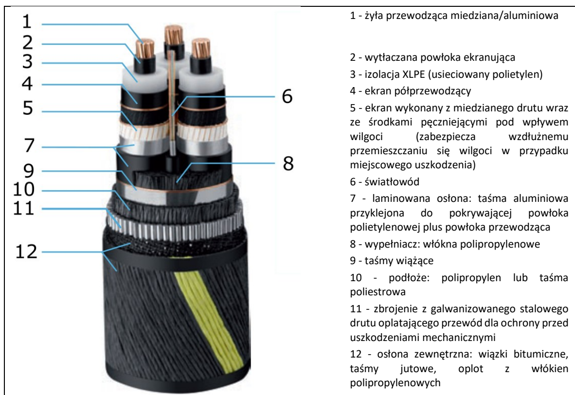
Rysunek 3.5. Budowa przykładowego podmorskiego kabla elektroenergetycznego najwyższych napięć (źródło: opracowanie własne na podstawie nexans.com)
