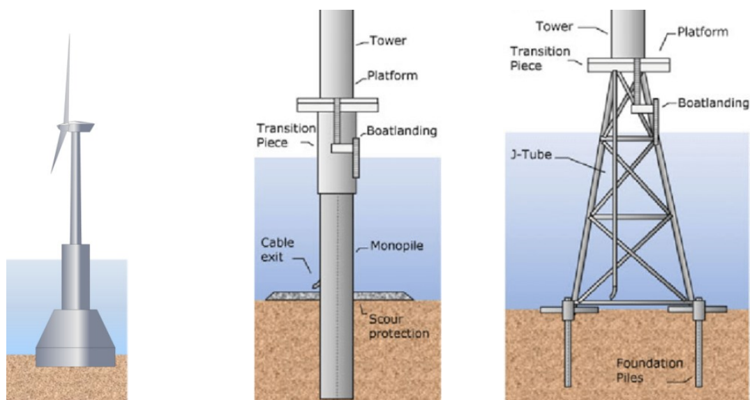
Rysunek 3.4. Poglądowe rysunki poszczególnych typów fundamentów (od lewej): grawitacyjny; monopłowy; kratownicowy (źródło: https://www.obayashi.co.jp/chronicle/130th/en/archives/chapter4_1_5.html# oraz: https://www.researchgate.net/figure/Three-types-of-turbine-foundations-Monopile-a-jacket-b-and-gravity-based-c_fig2_315874967 )
