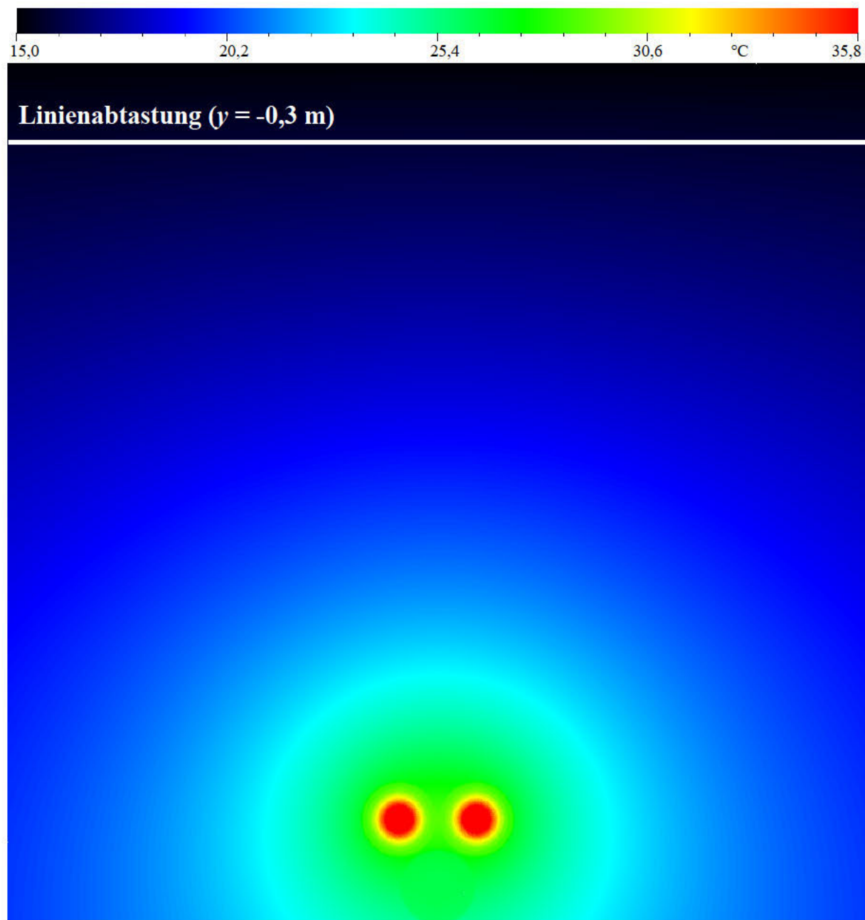
Abb. 26: Temperaturverteilung im stationären Vorzustand, FEM-Berechnung
