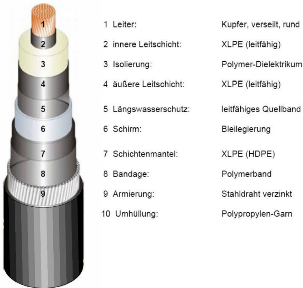
Abb. 2: Aufbau eines Einleiter-Hochspannungs-Gleichstrom-Seekabels [ABB2020]
