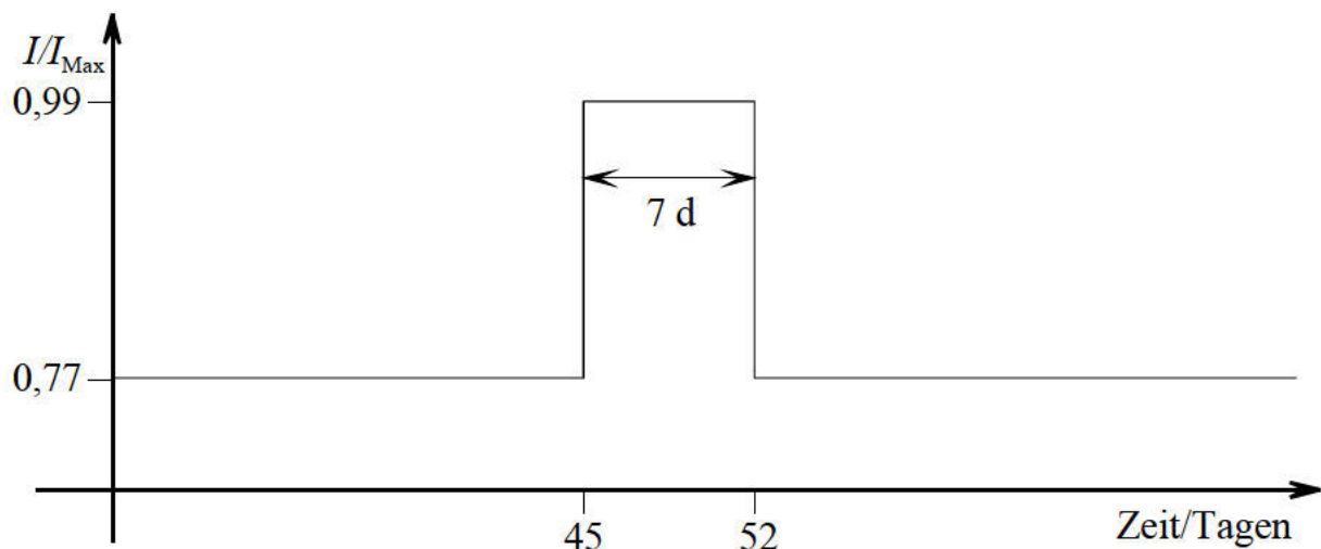
Abb. 1: Strombelastungsprofil für Offshore Windparks
